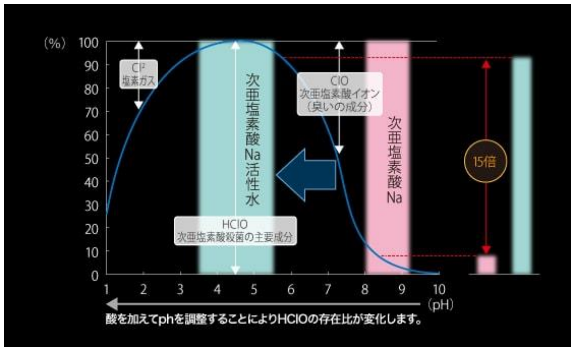
図：次亜塩素酸の存在率と pH
